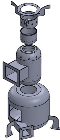
Gambar 2. a.Perancangan Tungku Si Badai dan b Proses Pembuatan
